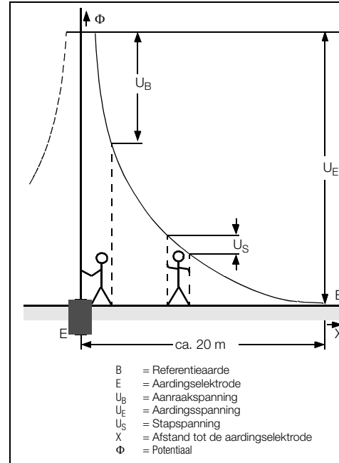
Plaatje 1 Aardoppervlakpotentiaelen en spanningen bij een onder stroom staande aardingselektrode
