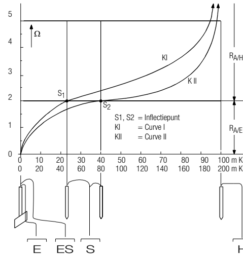
Plaatje 6 Meten van de aardingsweerstand van een verspreid aardingsysteem
