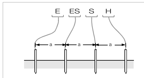
Plaatje 7 Meten van de bodemweerstand
